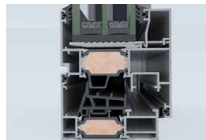
ELVIAL I 2 _ ΚΑΙΝΟΤΟΜΟΣ ΤΕΧΝΟΛΟΓΙΑ ΜΟΝΩΣΗΣ
